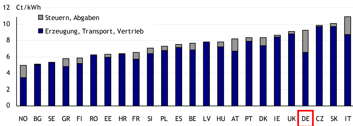
Abbildung 5 Europäische Industriestrompreise (Verbrauch von 70-150 GWh) in 2012 (1. Halbjahr)
