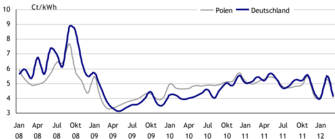
Abbildung 3 Börsenstrompreise (Spotmarkt Baseload, Monatsmittel) 2008 bis März 2012 in Deutschland und Polen
