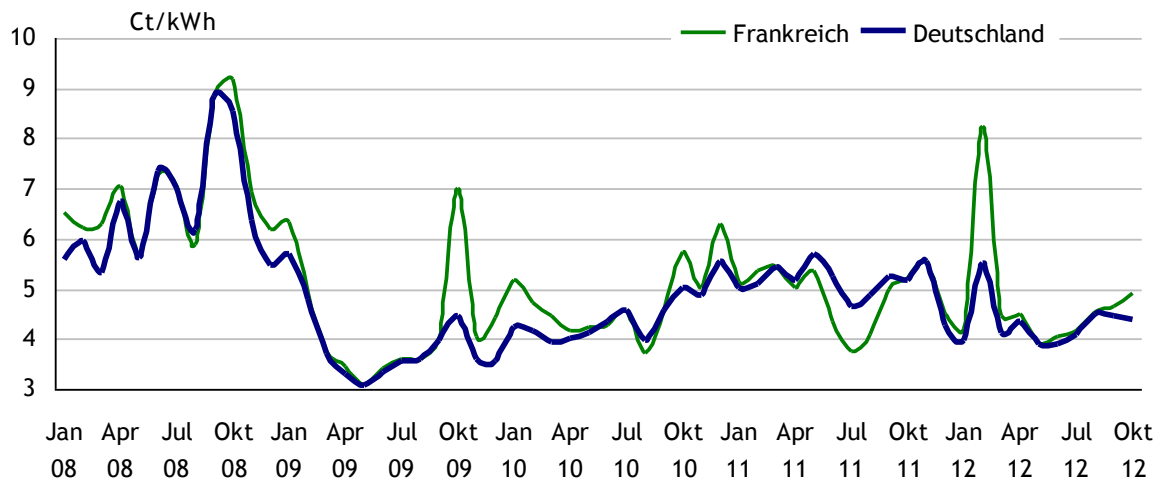
Abbildung 2 Börsenstrompreise (Spotmarkt Baseload, Monatsmittel) 2008-2012 in Deutschland und Frankreich
