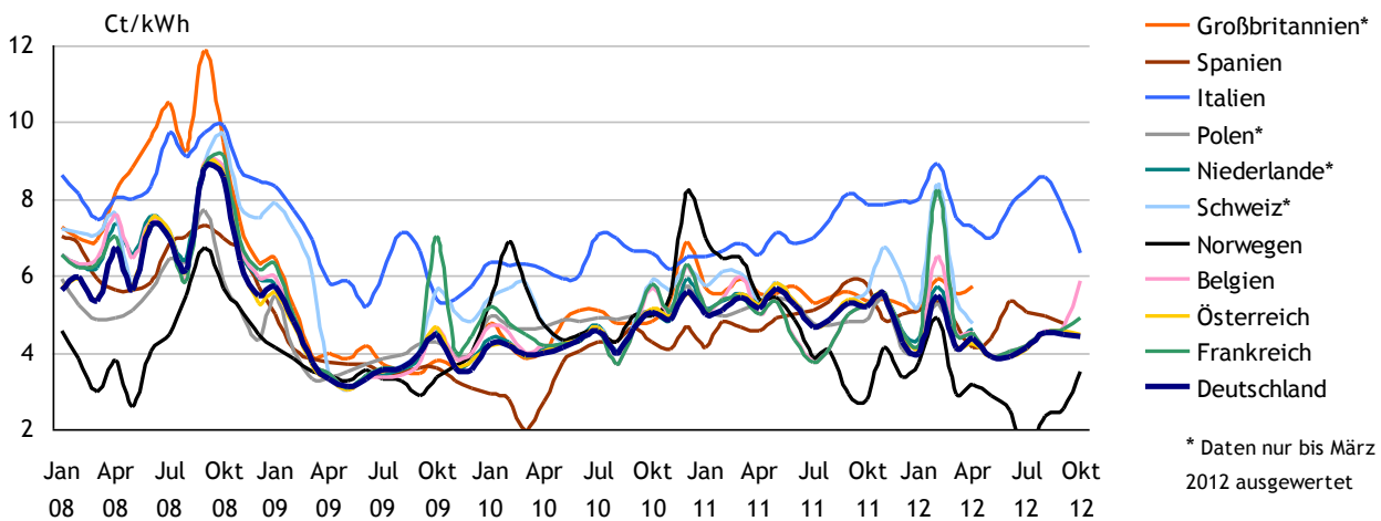
Abbildung 1 Börsenstrompreise (Spotmarkt Baseload, Monatsmittel) 2008-2012 im europäischen Vergleich
